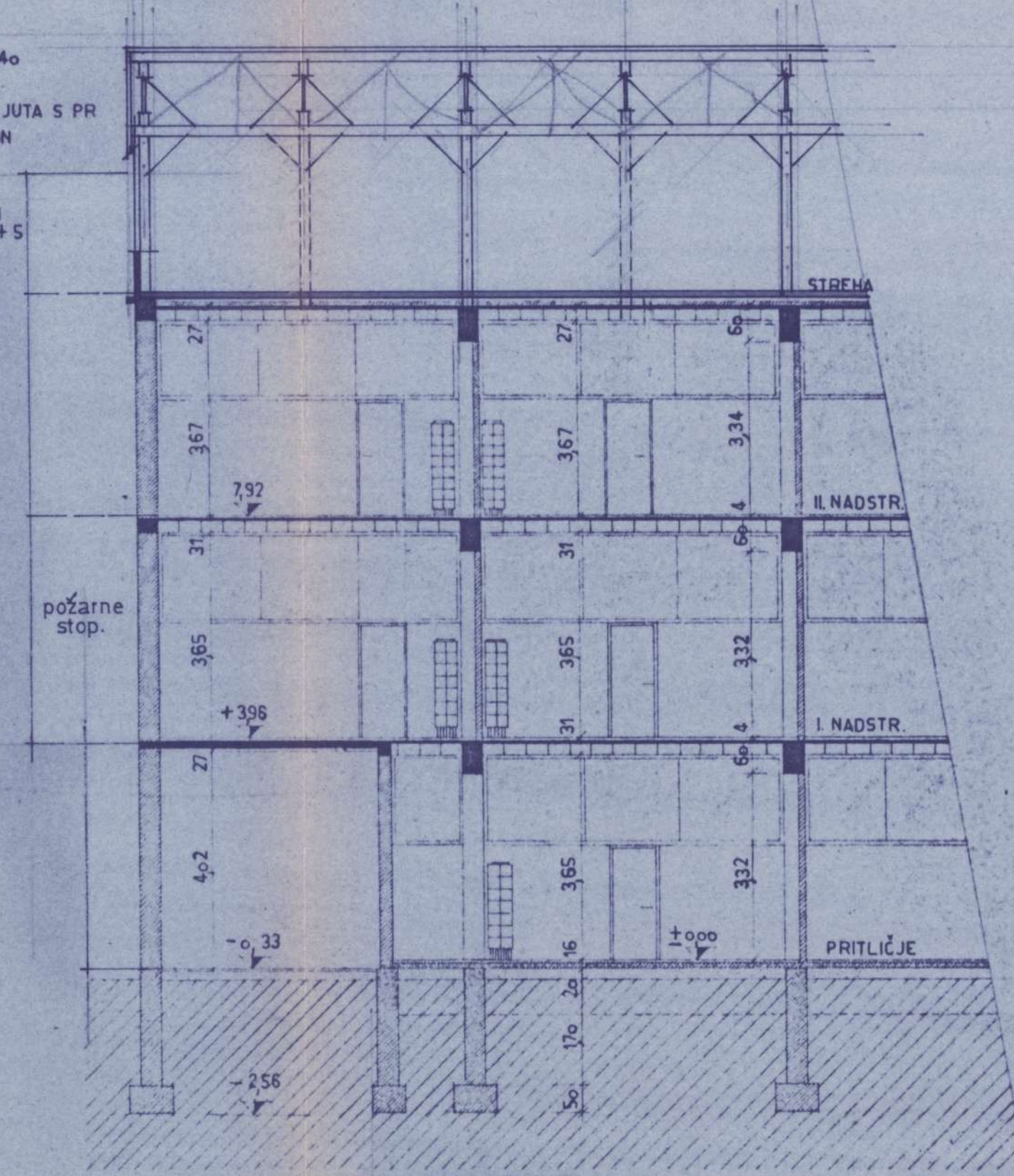
VZDOLŽNI PREREZ
