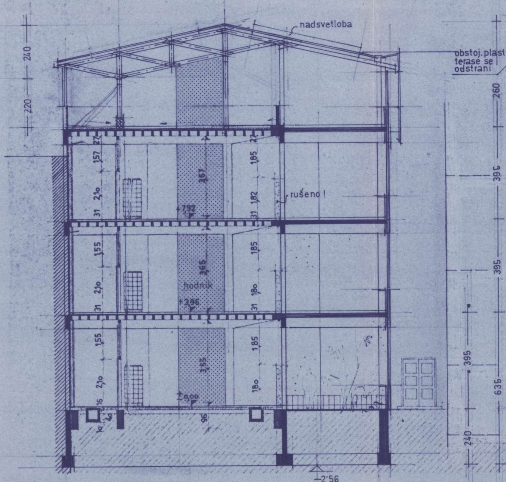
PREČNI PREREZ
