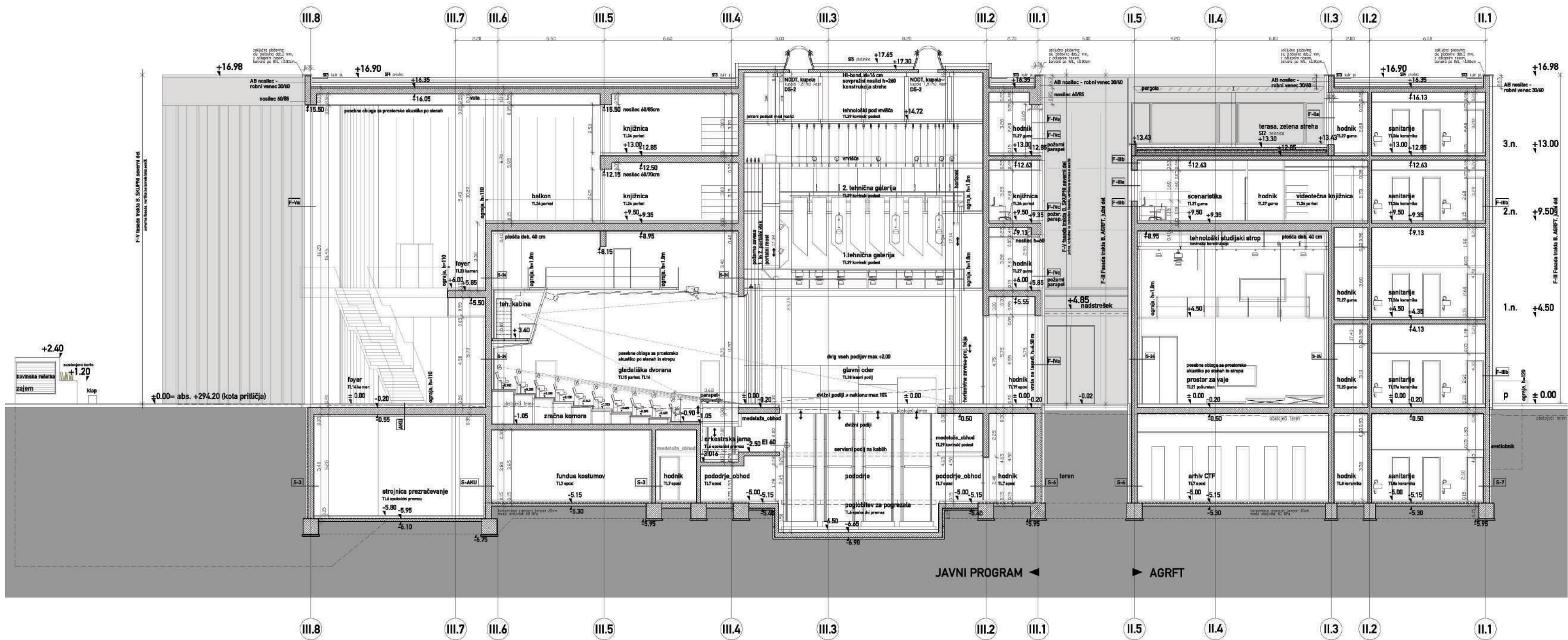
prerez D-D
